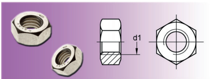
Sechskantmutter - Metall ~DIN 934 (~DIN EN ISO 4032)
