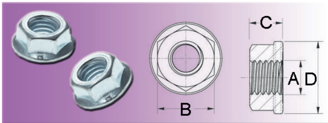
Sechskantmutter mit Flansch - Metall ~DIN 6923 ohne Sperrverzahnung (~DIN EN 1661)
