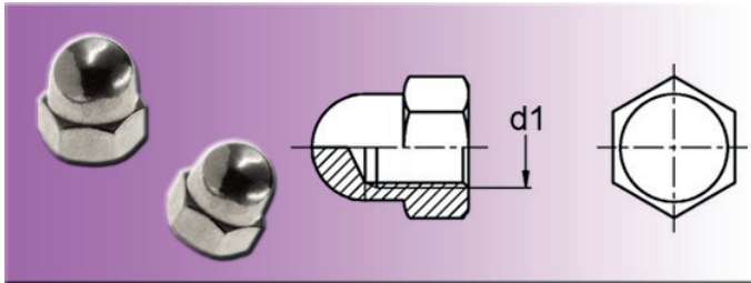
Hutmutter - Metall ~DIN 1587
