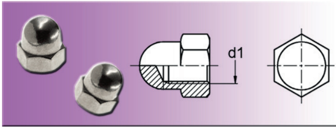
Hexagon cap nuts - metal ~DIN 1587
